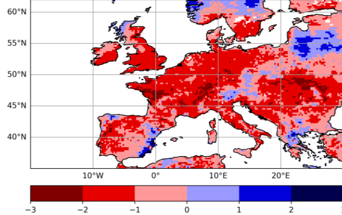
SWI layer 3 z-score (-), Aug 2022
